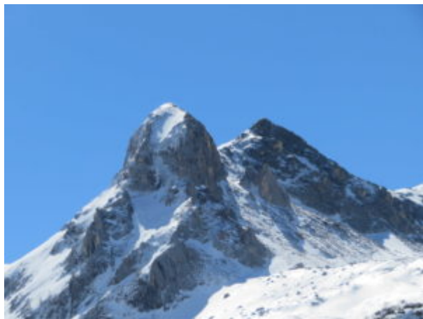
Rocca dell'Inferno
